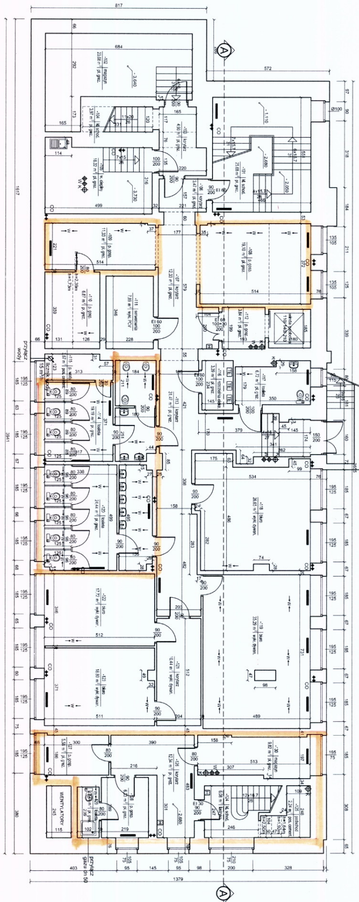
RZUT PIWNICY skala 1:100
